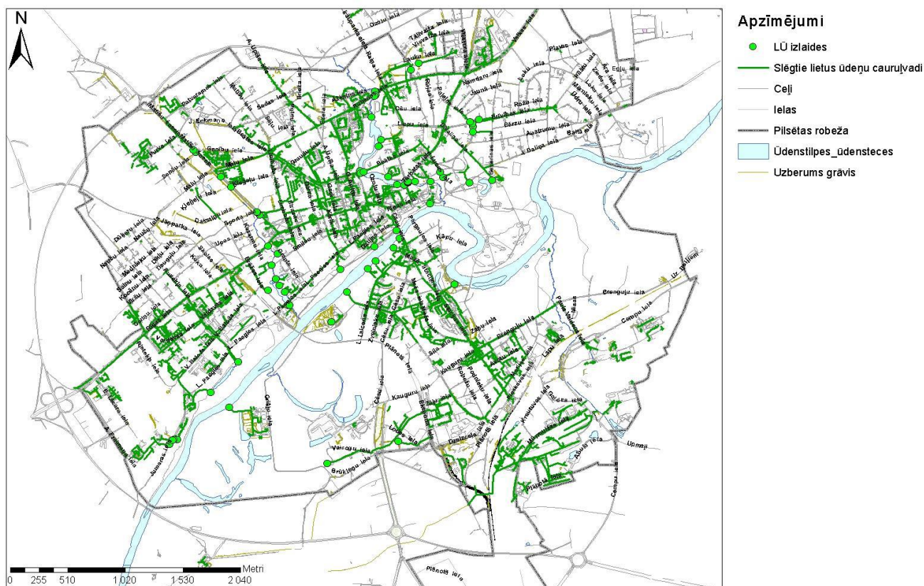
Shēma centralizētās lietus ūdeņu savākšanas sistēmai Valmieras pilsētā. SIA "Valmieras ūdens" GIS datu bāze, 2015
