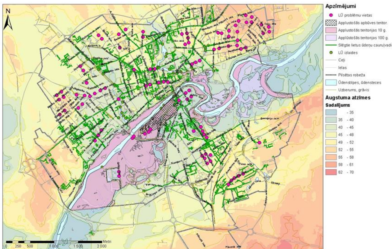
Esošās situācijas lietus ūdeņu novadīšanā Valmieras pilsētā shēma. (R.Višņevskas izstrādāts pēc SIA „Valmieras ūdens”, 2016; LĢIA, 2016; Valmieras pilsētas pašvaldība, 2016)
